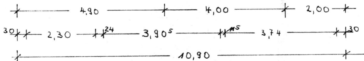
Obergeschoss
